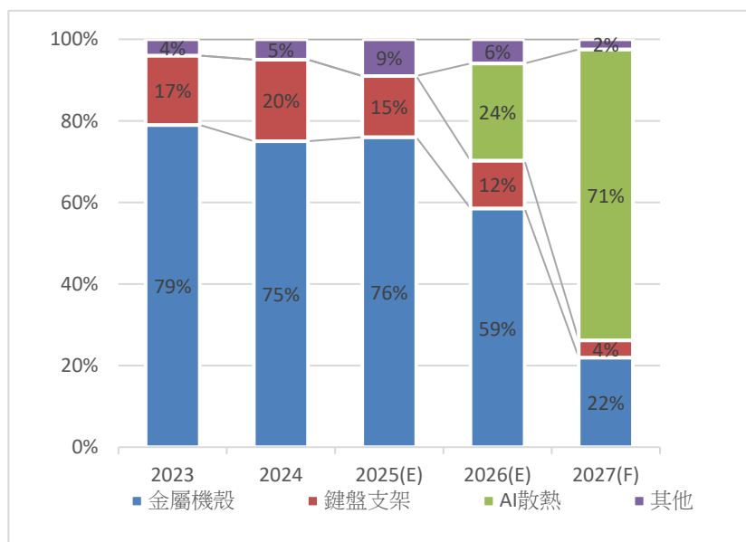
圖一、濱川產品組合營收
